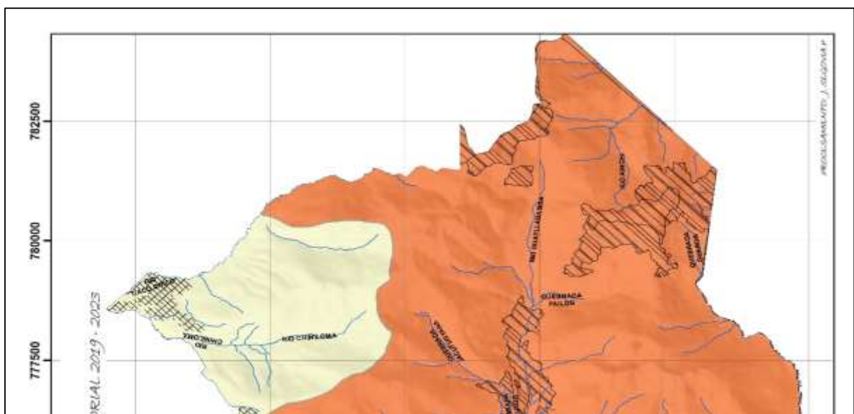
Imagen 9.2. Ecosistemas
