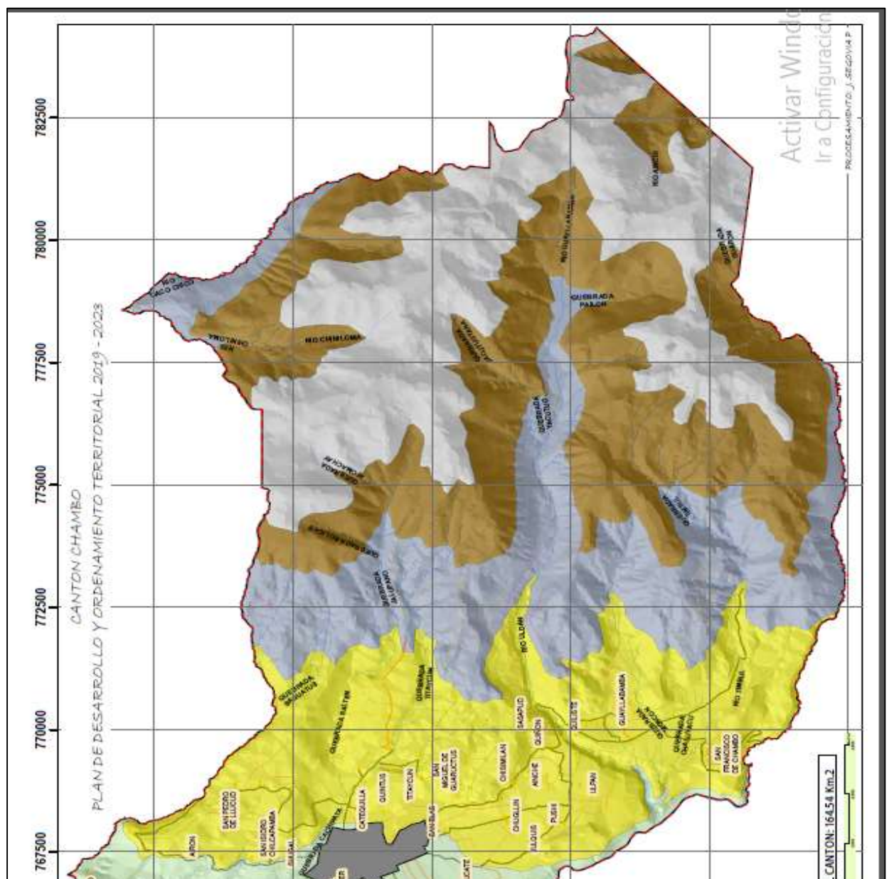
Imagen 12.2. Pisos altitudinales
